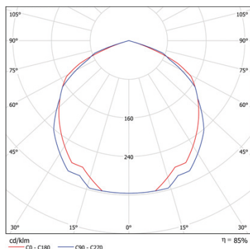
Lichtstärkeverteilung (bei 30W)
