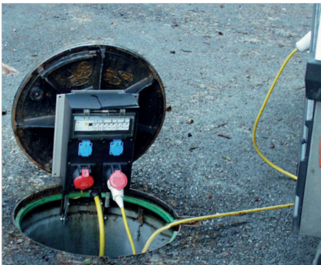
Unterflurverteiler für die Anspeisung von Kühlfahrzeugen.
