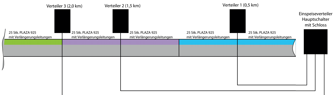
Anspeisungsschema
