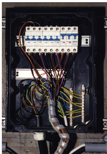
Plabutschunnel - selbst bei hoher Luftfeuchtigkeit und starken Temperaturschwankungen keine Bildung von Kondenswasser im Innenbereich des Verteilers
