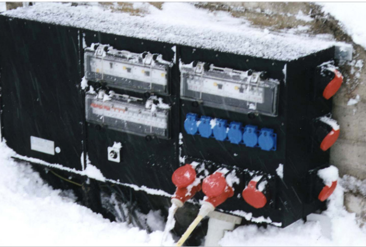
Eventverteiler mit 4x240mm² - auch im gesteckten Zustand kein Eintritt von Wasser oder Feuchtigkeit
