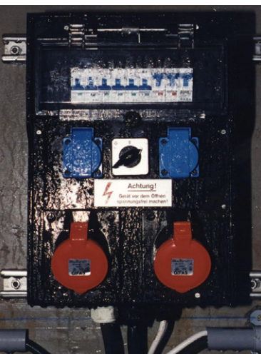
Plabutschunnel - selbst bei hoher Luftfeuchtigkeit und starken Temperaturschwankungen keine Bildung von Kondenswasser im Innenbereich des Verteilers
