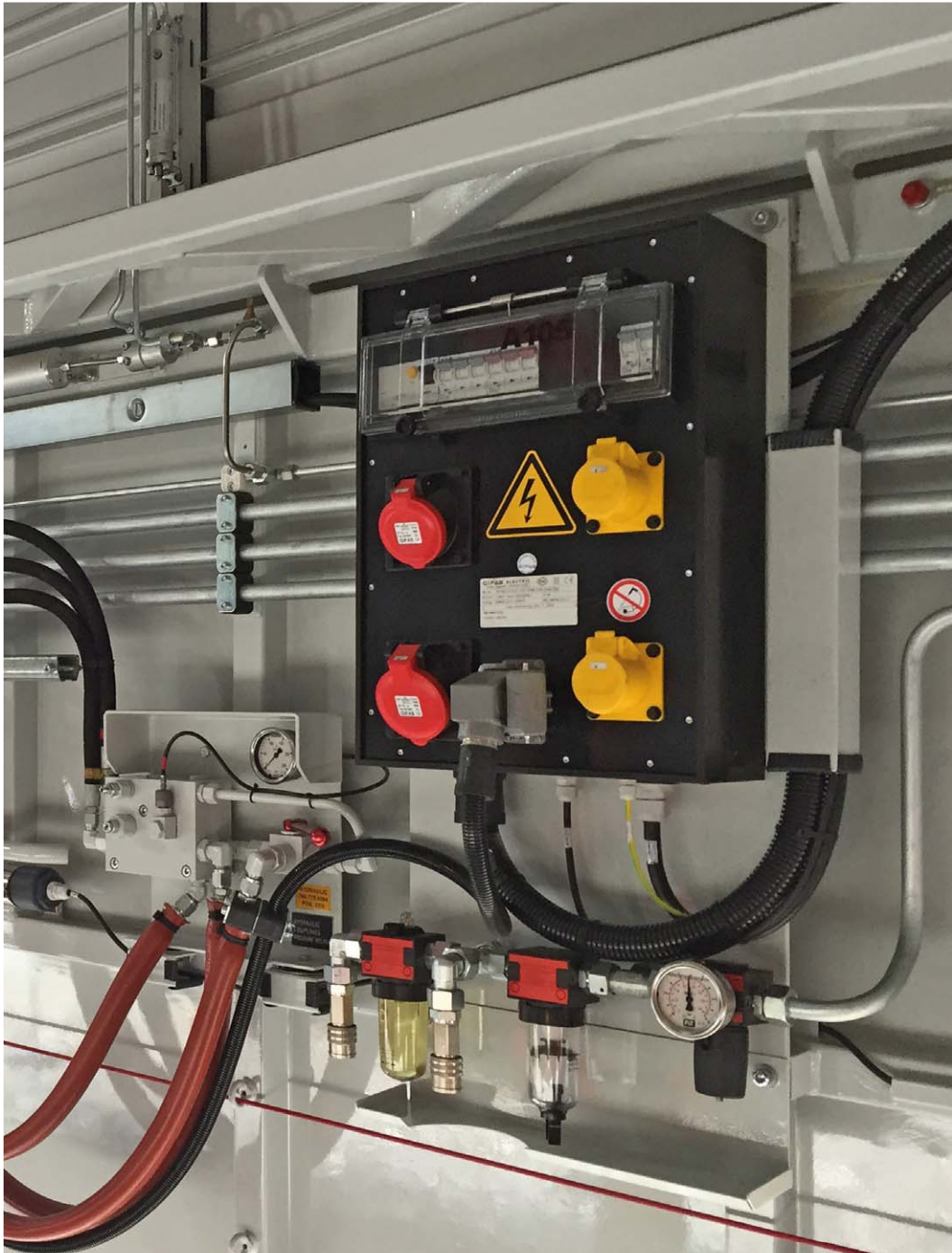
Vollgummi Wandverteiler
