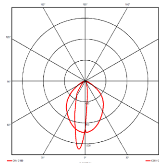
Lichtstärkeverteilung
