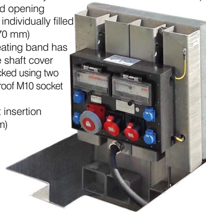
PIAZZA 700 max. pre-fuse 125A
